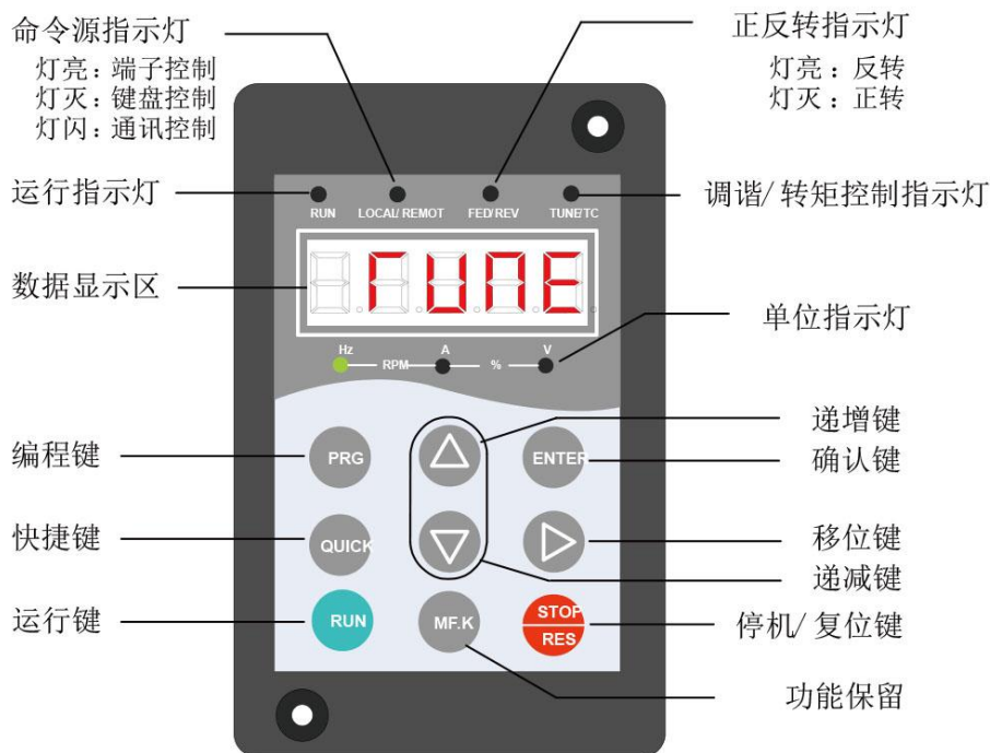
图 7-2 汇川变频器操作面板
