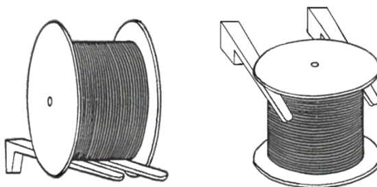
图 8-21 钢丝绳错误装卸
