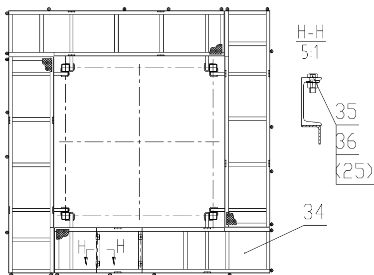
下平台布置图
