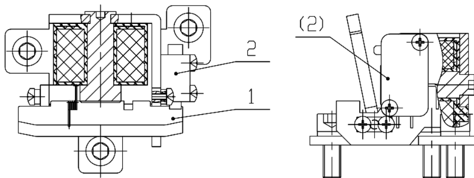
图 8-12 电磁铁组件
