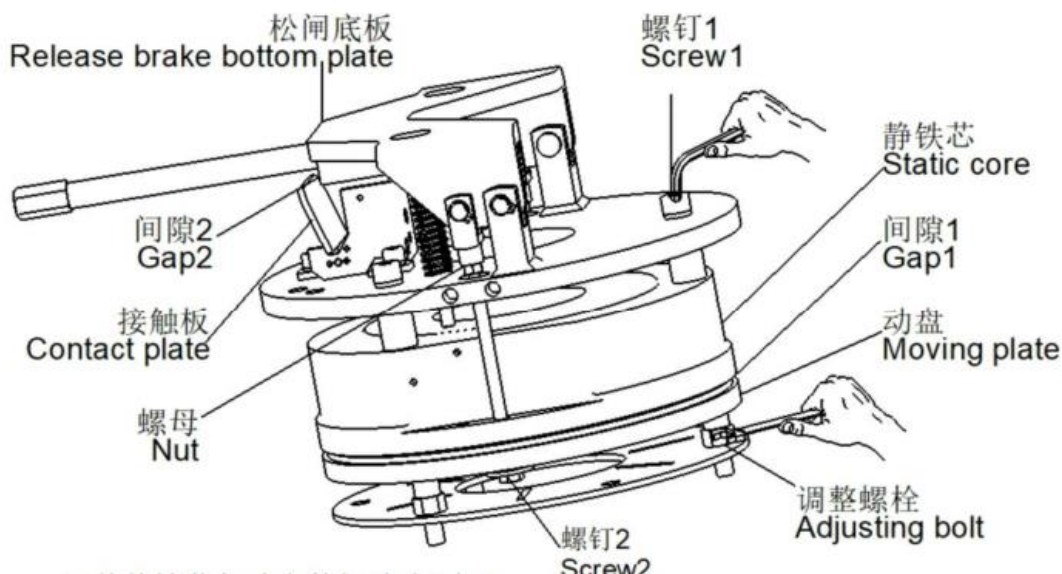
图 8-13 调间隙示意图
