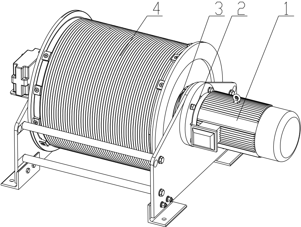
1-电机 2-联轴器 3-减速机 4-卷筒
