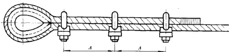
图 8-29 钢丝绳夹间的距离
