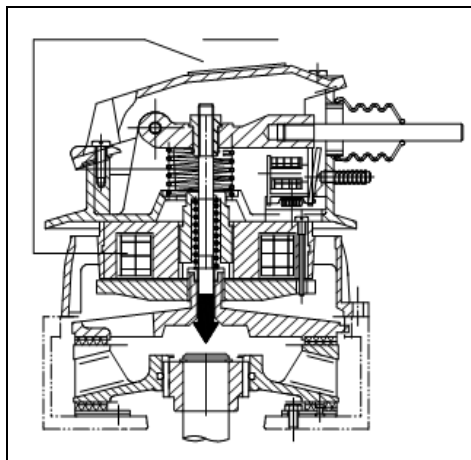
图 8-a 制动状态
