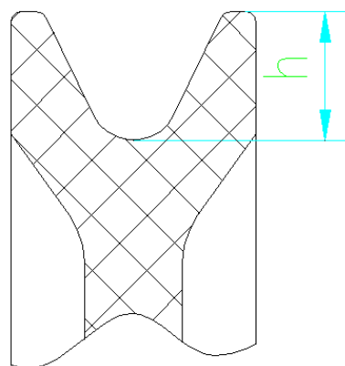
图 8-b 绳槽深度检测
