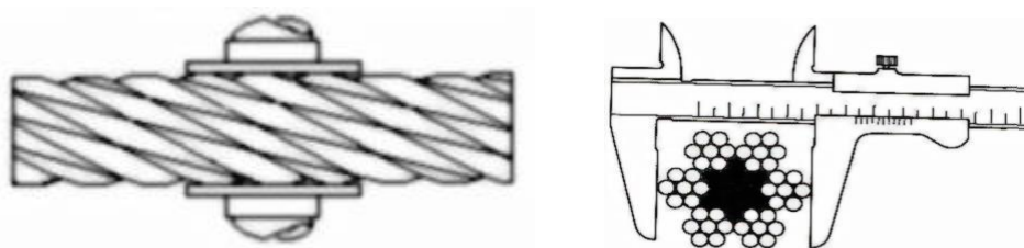
图 8-18 钢丝绳直径检测
