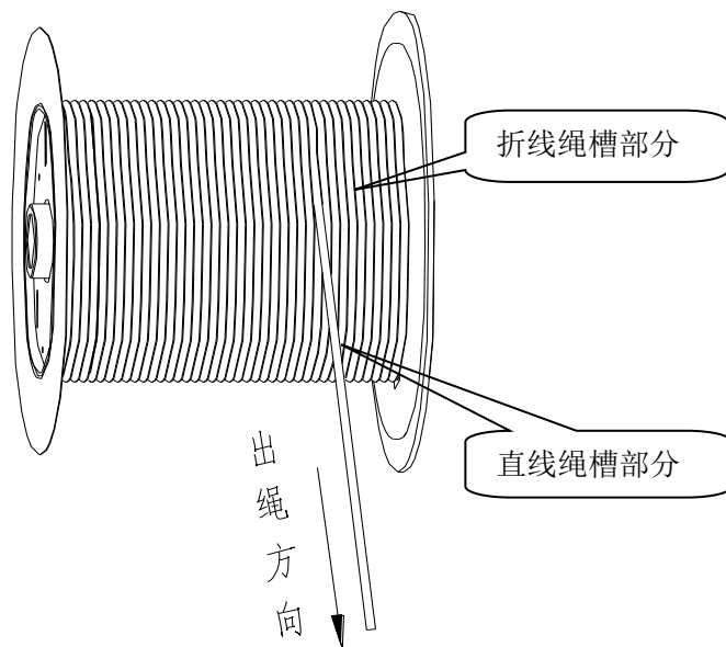
图 8-3 卷筒结构图
