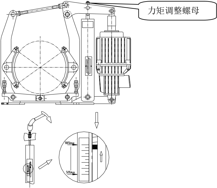
图 8-4 制动力矩的调整
