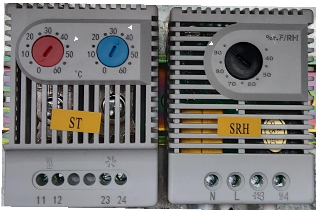
图 8-a 温度开关
