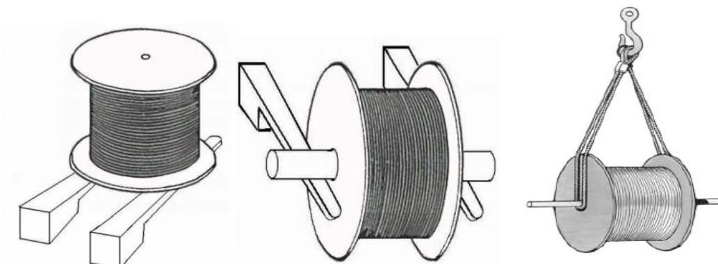
图 8-20 钢丝绳正确装卸
