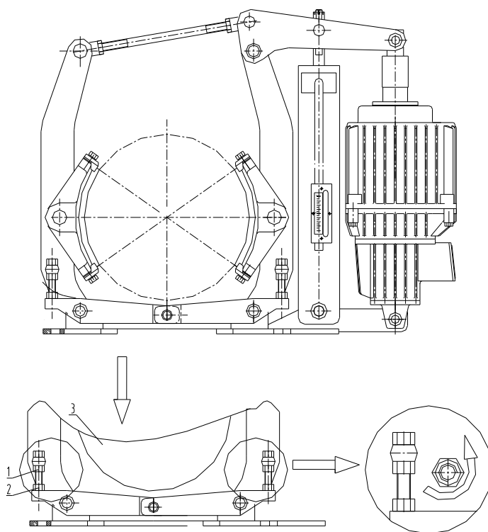
1-锁紧螺母2-锁紧螺母3-制动轮
