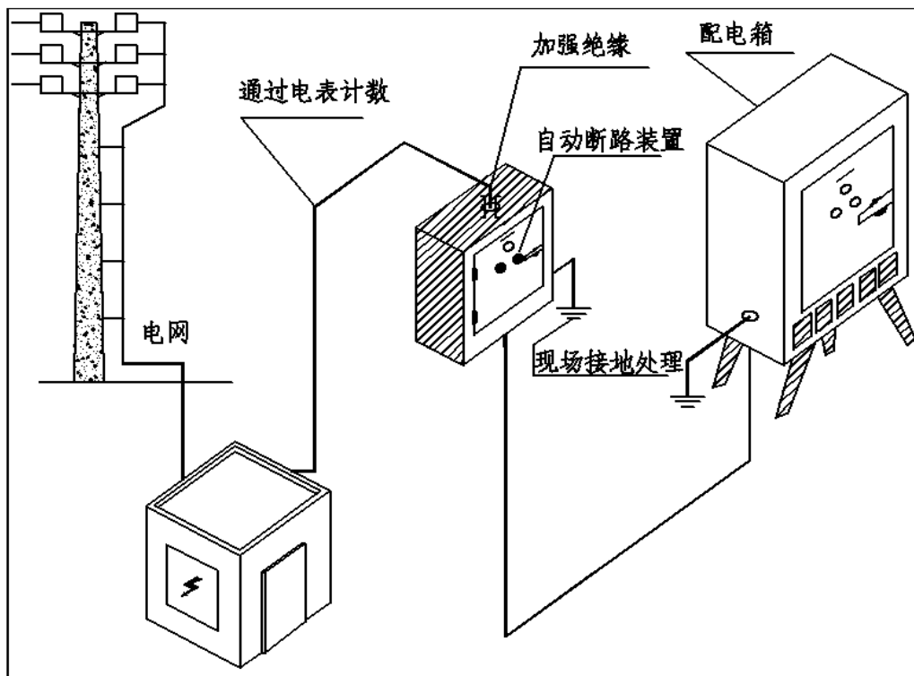
图 7-1 工地电源布置图
