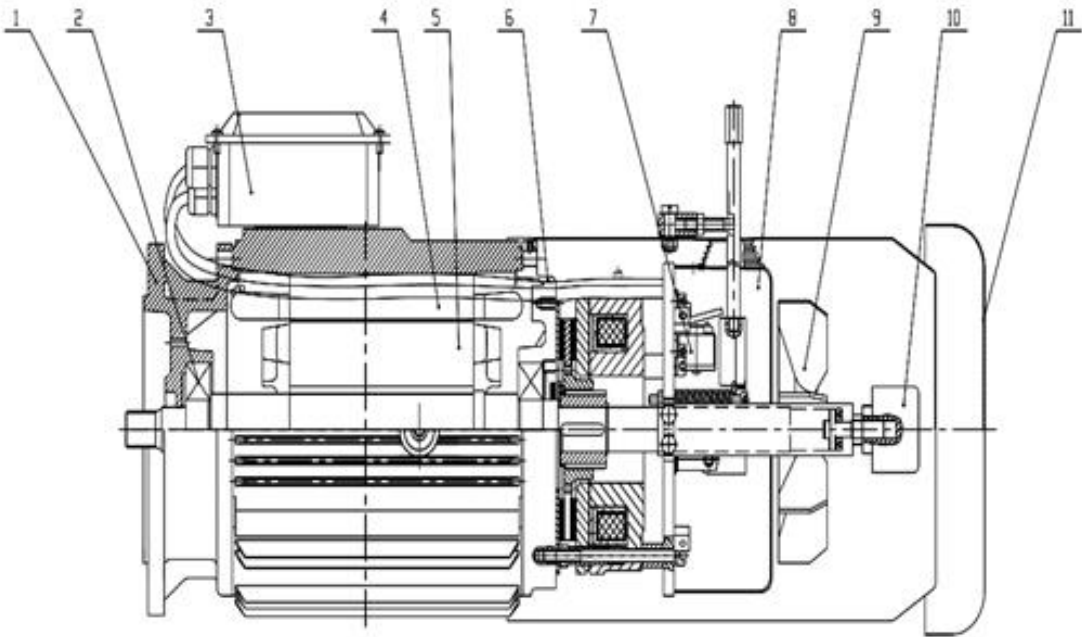
图 8-10 YTRVF 系列 F1 带风标制动器塔机用变频电动机结构图
