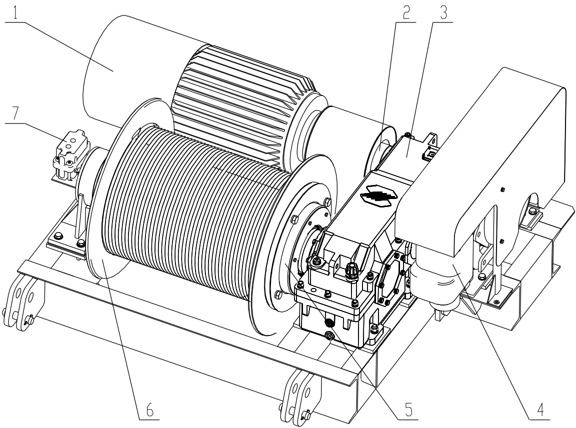
1-电机 2-联轴器 3-减速机 4-制动器 5-齿形接盘 6-卷筒 7-高度限位器
