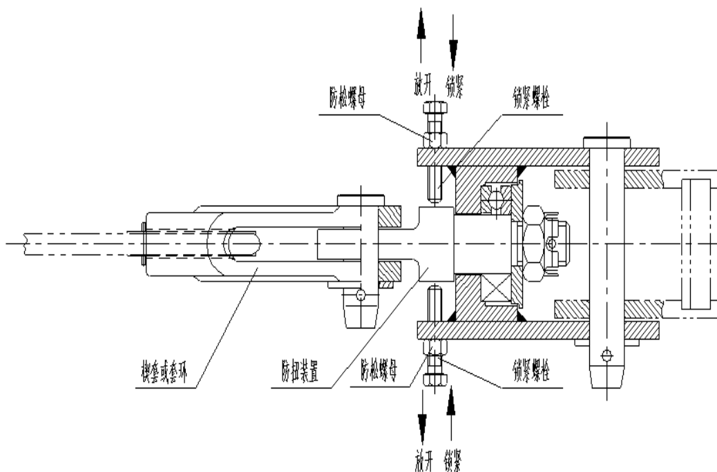
图 8-27 防扭装置
