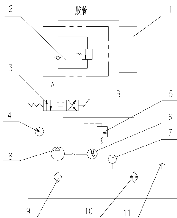
图 8-14 液压系统接管示意图
