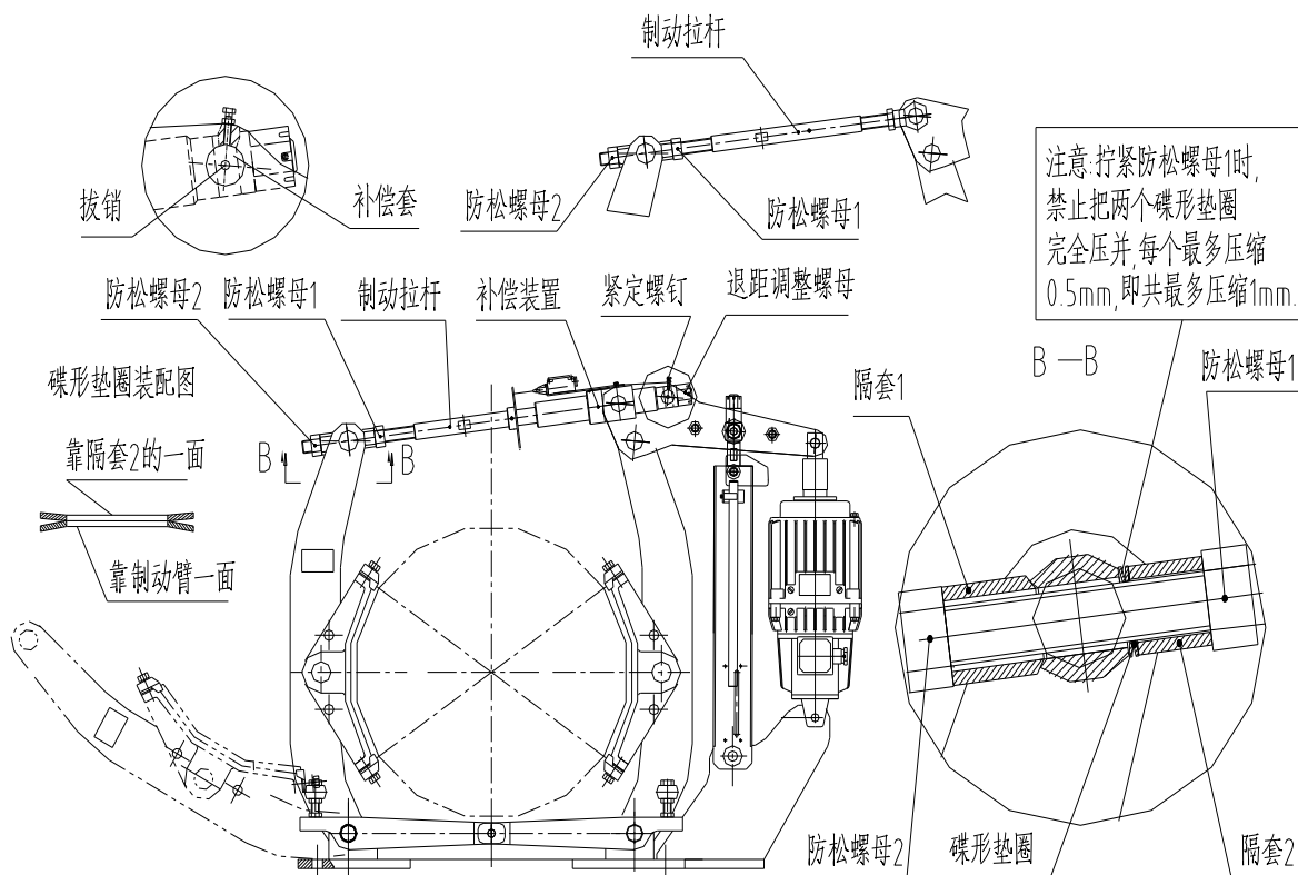
图 8-3 制动器结构
