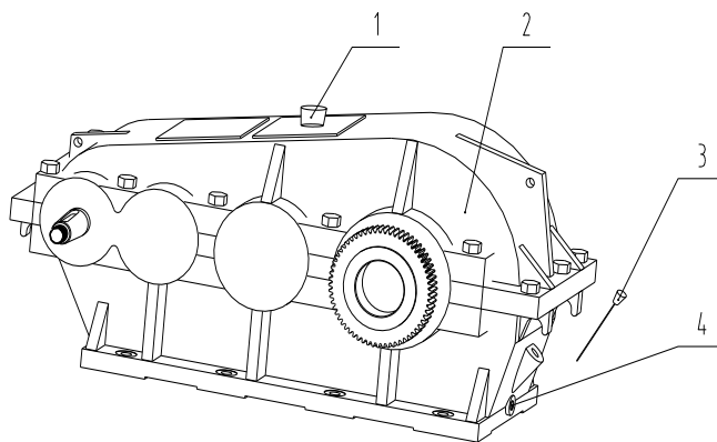
1.进油口 2.箱体 3.油尺 4.排油堵
