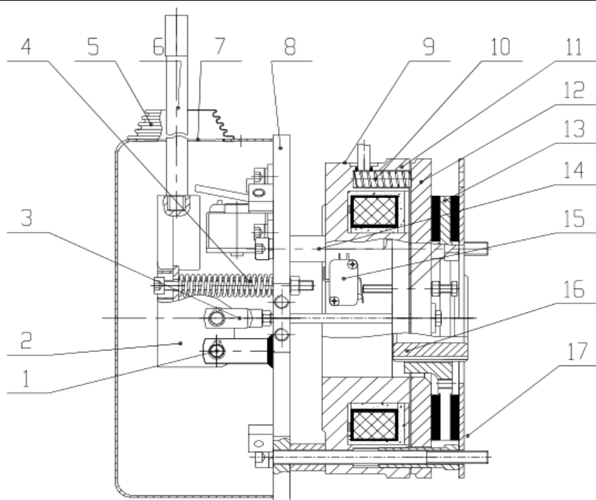
图 8-11 风标制动器结构图
