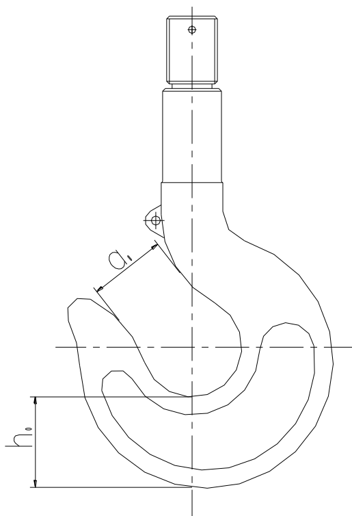
图 8-38 吊钩的开口度和磨损
