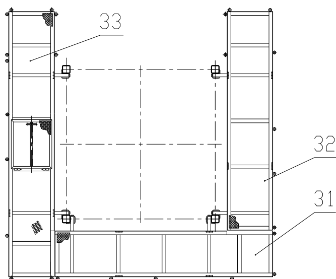
上平台布置图
