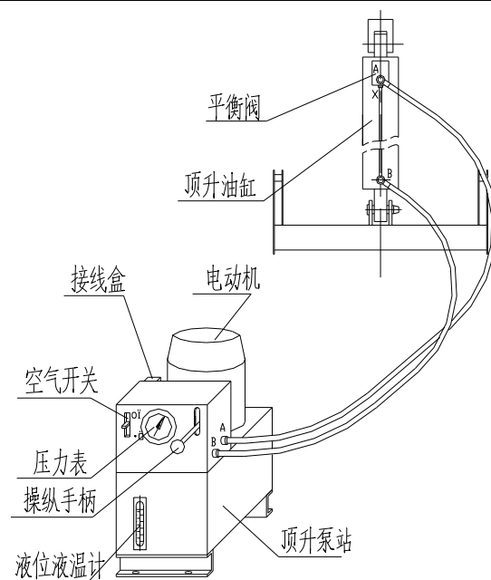
图 8-14 液压系统接管示意图
