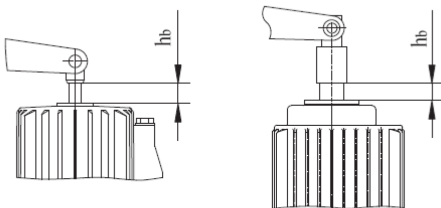
图 8-5 瓦块退矩的调整
