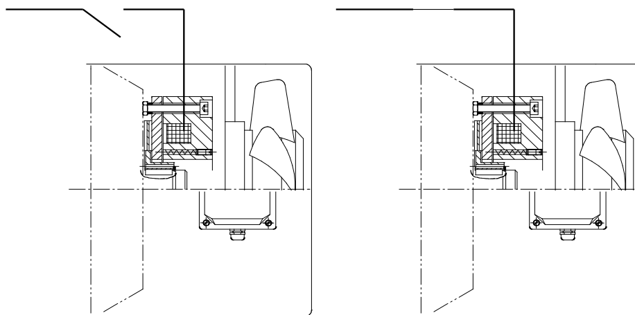
图 8-7a 电磁制动器制动
