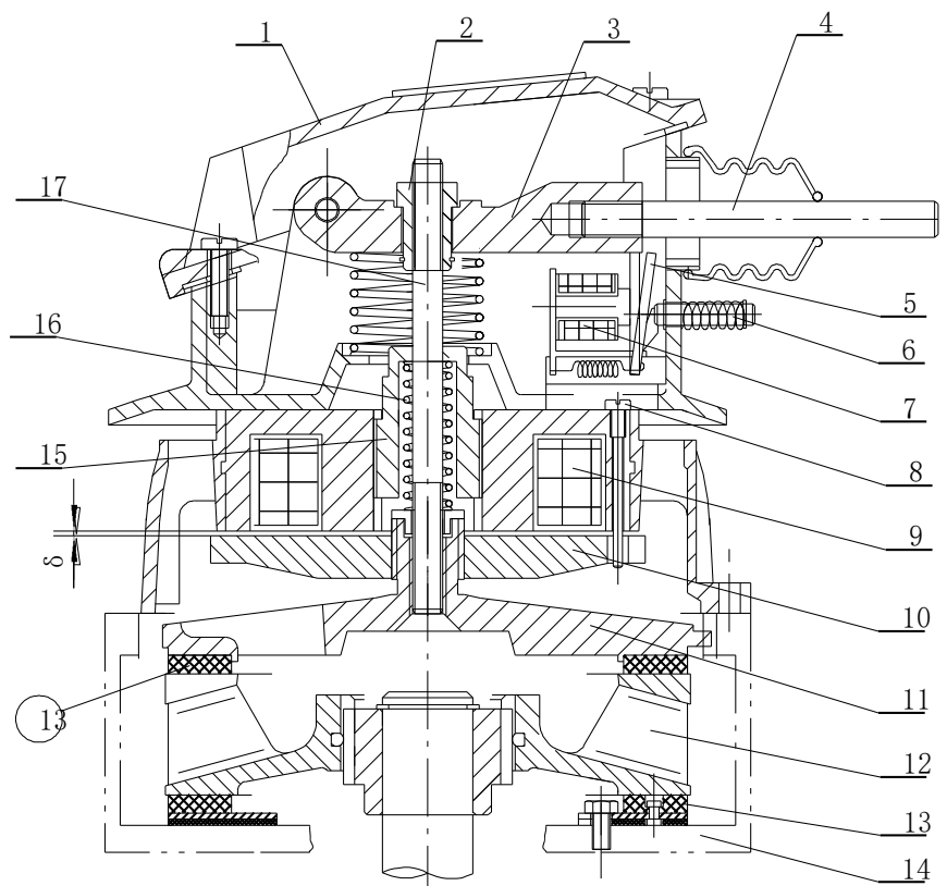
图 8-19 制动器结构图
