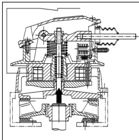
图 8-b 松开状态
