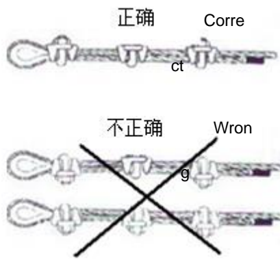
图 8-28 钢丝绳夹的正确布置方法
