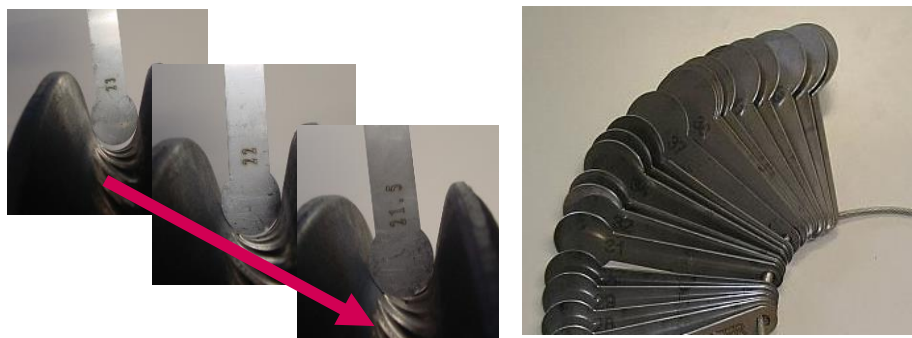
图 8-19 滑轮槽圆弧半径检测示例
