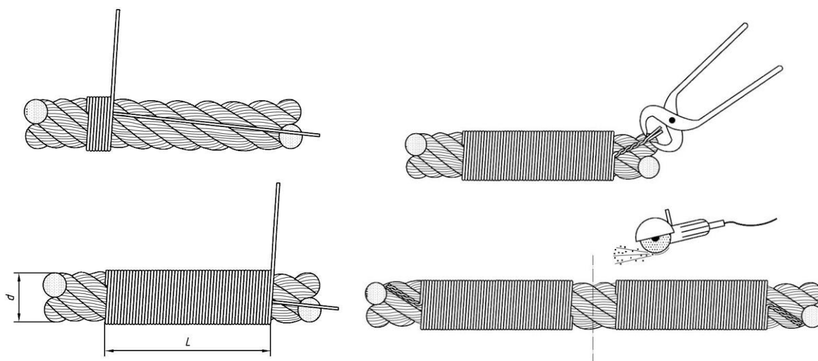
图 8-17 钢丝绳切断前的准备( L \geq 2d )
