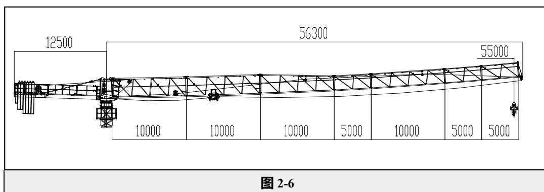
3) 50m臂长塔机上半部外形尺寸
