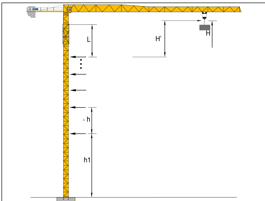
图 4-100 塔机附着示意图
