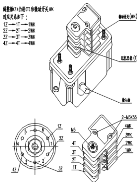
图 4-86 变幅限位器图
