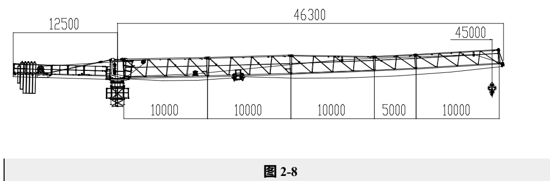
5) 40m臂长塔机上半部外形尺寸
