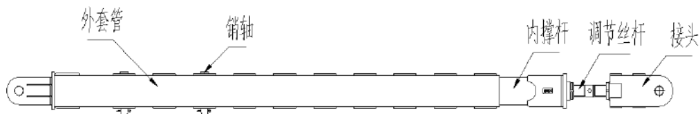
图 4-95 附着撑杆
