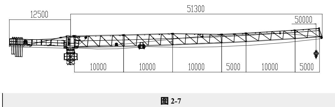
4) 45m臂长塔机上半部外形尺寸
