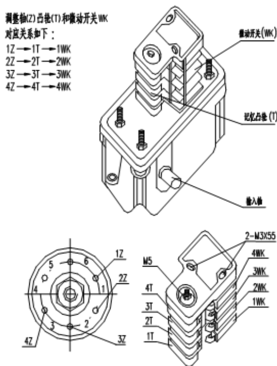
图 4-85 回转限位器图
