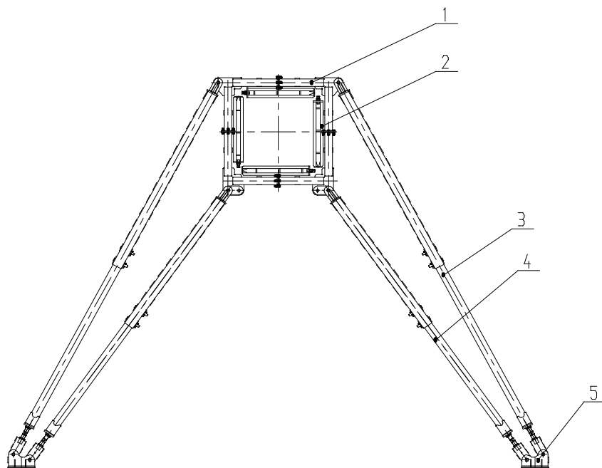
1-附着框 2-内撑杆 3-撑杆A 4-撑杆B 5-耳座
