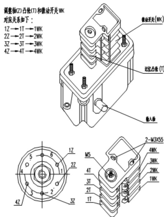
图 4-84 起升限位器图
