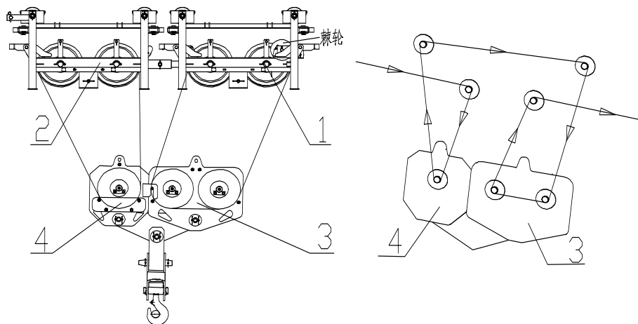
图 4.19-4 安装和绕绳示意图
