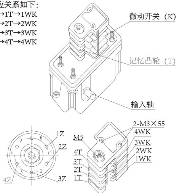
图 4.23-3 起升限位器图
