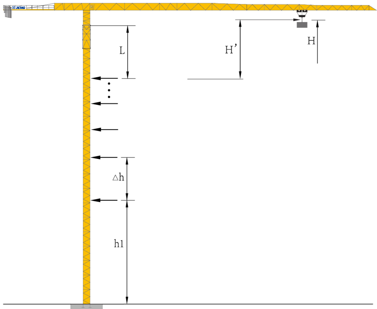
图 4.25-5 塔机附着示意图
