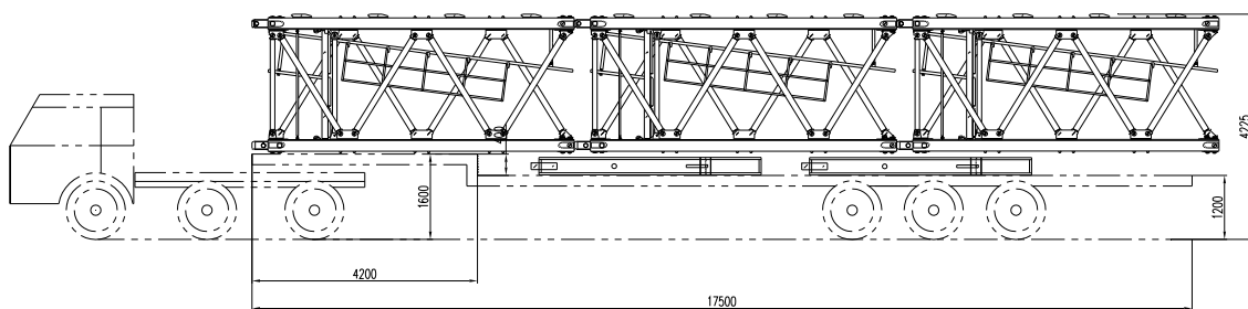
第八车：3 节 F88BC 标准节、2 块 4750 平衡重。
