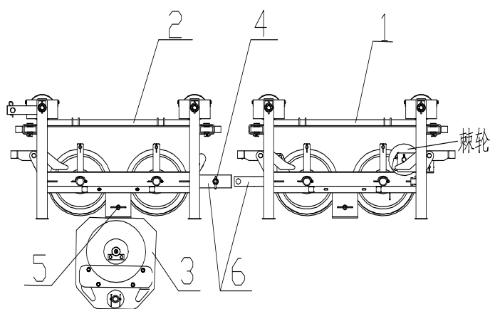
1-主小车 2-副小车 3-副吊钩 4-销轴 a 5-销轴 b 6-连接座 a
