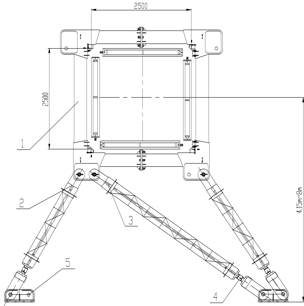
1-附着框 2-撑杆 I 3-撑杆 II
