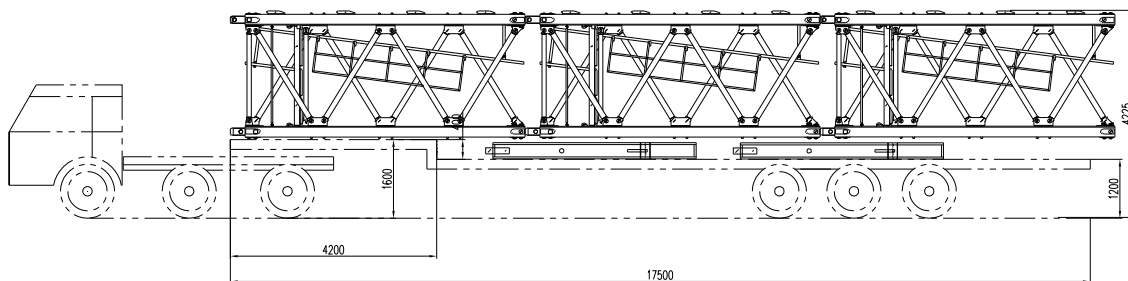
第七车：F89QC 加强节、2 节 F88BC 标准节、2 块 4750 平衡重。
