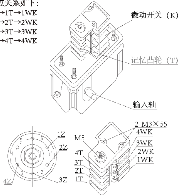
图 4.23-4 起升限位器图
