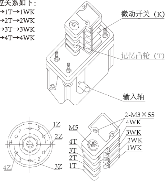
图 4.23-5 变幅限位器图
