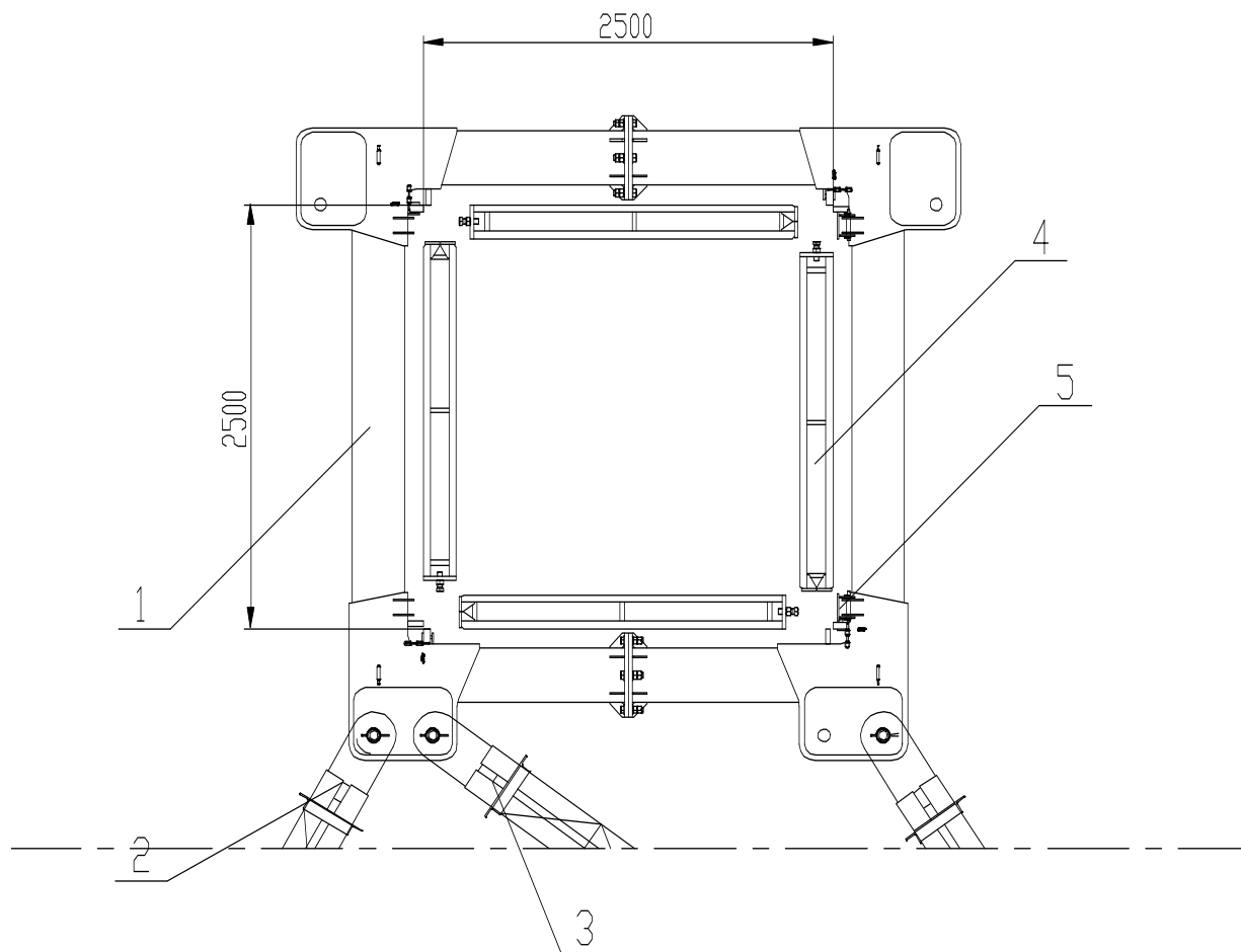
1-环梁 2-撑杆 I 3-撑杆 II 4-内撑杆 5-踏步吊耳
