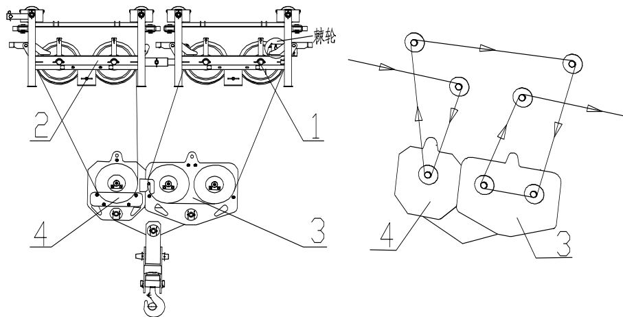
1-主小车 2-副小车 3-主吊钩 4-副吊钩
