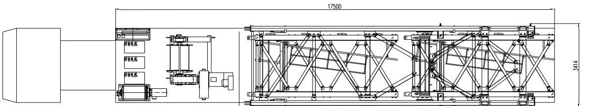
第六车：起重臂臂节3、起重臂臂节4、起重臂臂节5、起重臂臂节6、特殊节横梁、销轴箱、特殊节整体。
