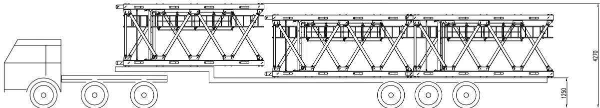
第四车：加强节整体×2、基础节整体。
