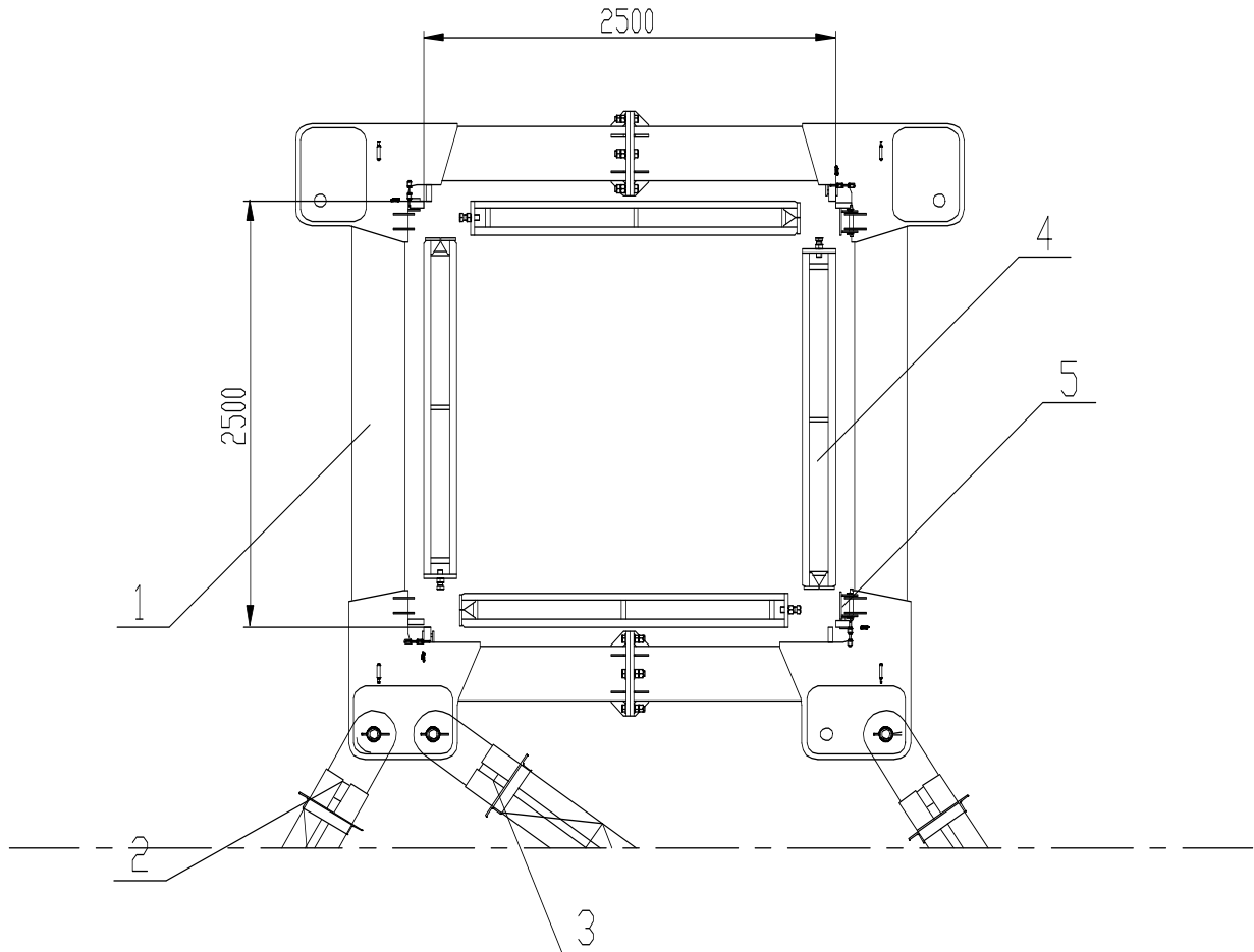
1-环梁 2-撑杆 I 3-撑杆 II 4-内撑杆 5-踏步吊耳
