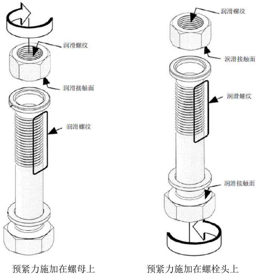
图 4.1-2 连接螺栓接触表面的润滑
