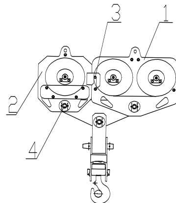
1-主吊钩 2-副吊钩 3-销轴 c 4-销轴 d
