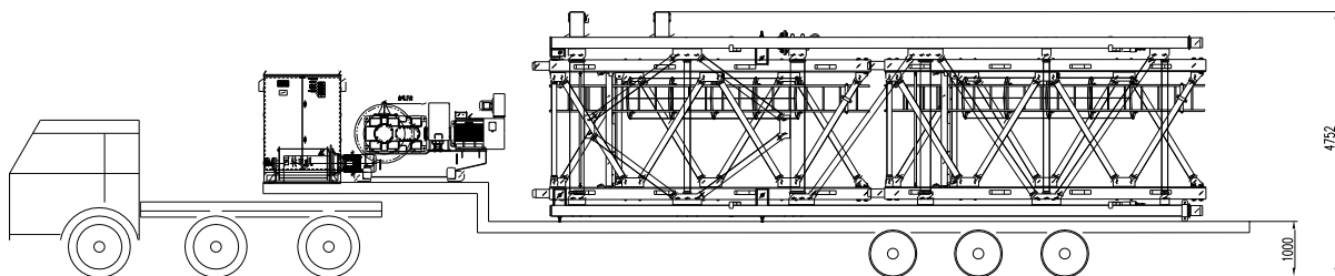
第五车：爬升架结构整体、标节整体×2、电控柜、变幅机构、回转电机、起升机构。
